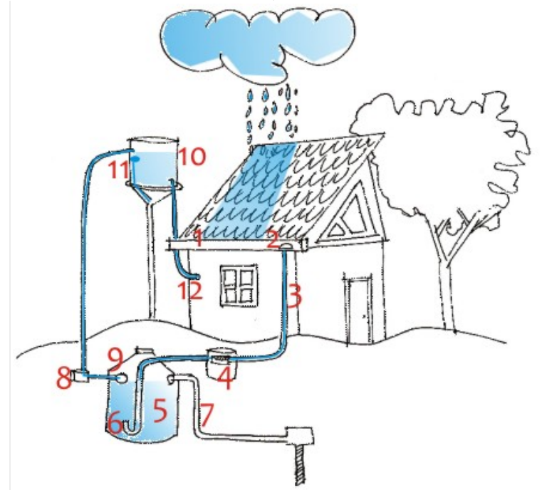
Esquema demonstrativo de um sistema típico de aproveitamento da água da chuva
